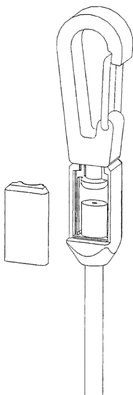
【内部の構造を説明するための参考斜視図】
