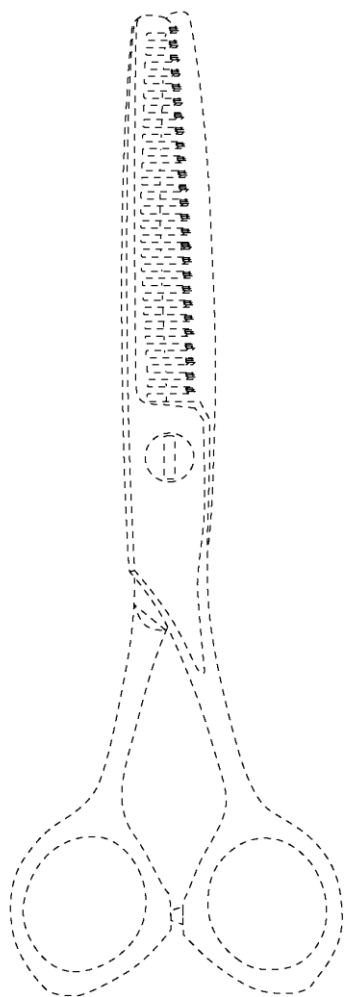
【A－A部分拡大図】
