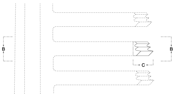
【背面図】
