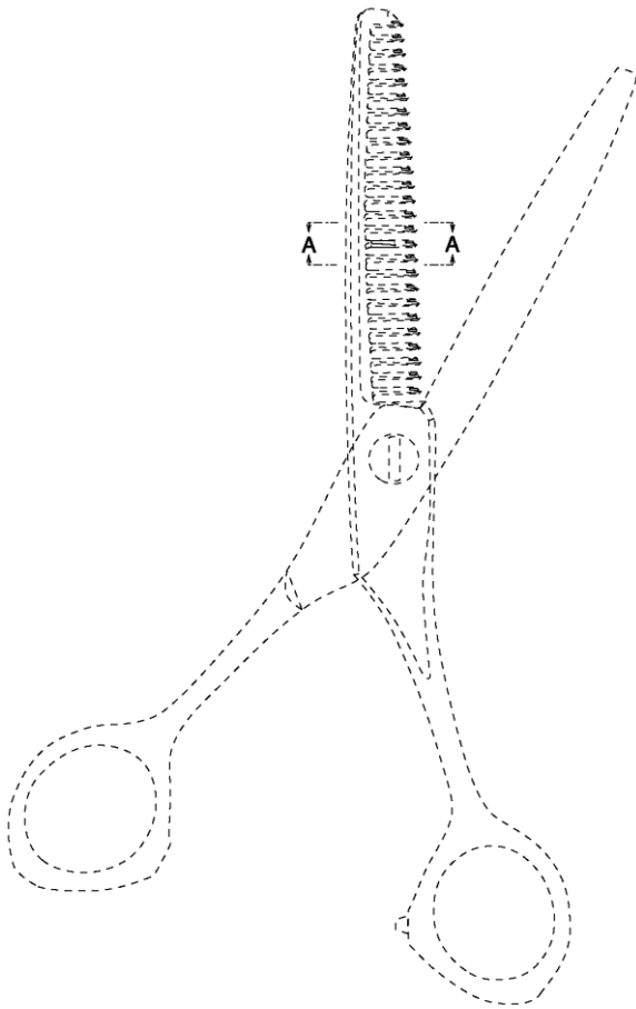
【開いた状態の正面図】
