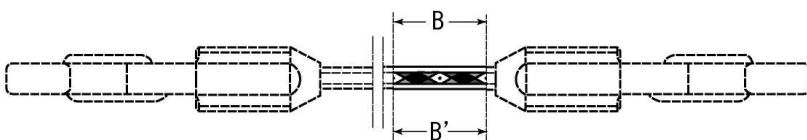
【B－B'部分拡大正面図】
